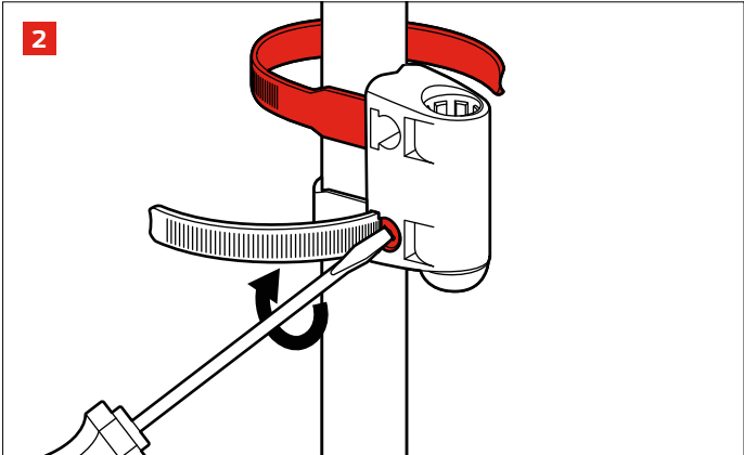
2 Die Laschen durch die Halterung führen und mit einem Schraubenzieher festziehen. Inserting the straps through holder and tighten with a screwdriver.
